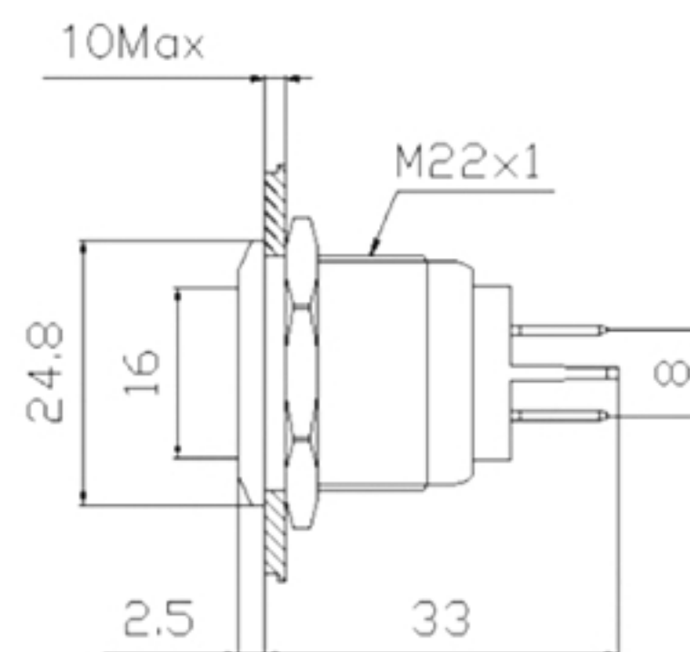
外形尺寸 Diameter
